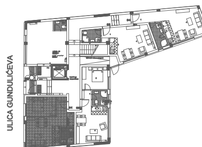
OSNOVA PRIZEMLJA
